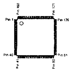
μPD77016GM-KMD (Q7101)
