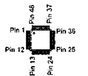
MB89133APFM (Q5035)
